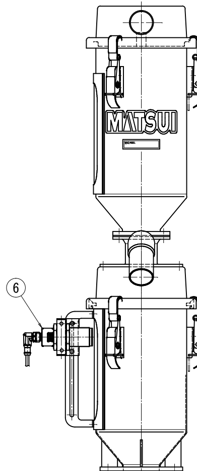
In case of EFECTOR mounting. エフェクター取付の場合
